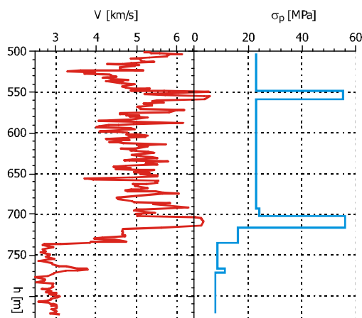
Obr. 8 Vztah rychlosti a pevnosti
