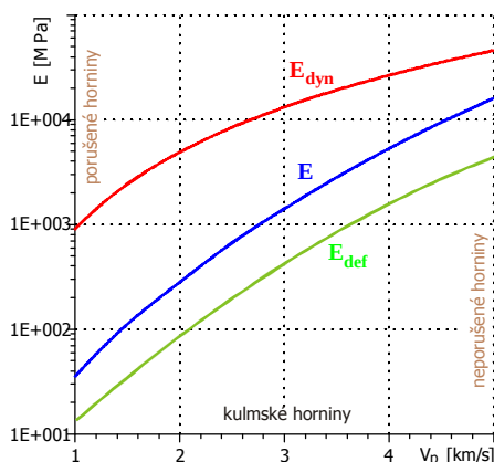
Obr. 7 Vazba V a E na Slezské Hartě (upraveno podle Mjuller, Novosad, 1986)
