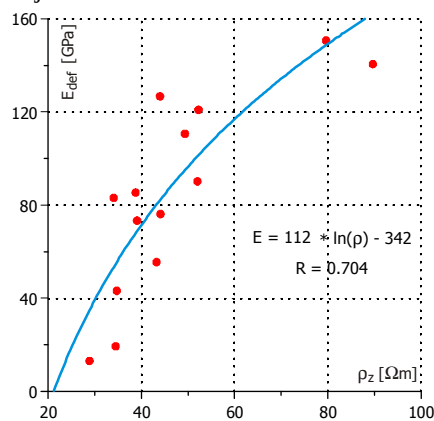
Obr. 12 E_{dyn} a \rho_z v násypu
