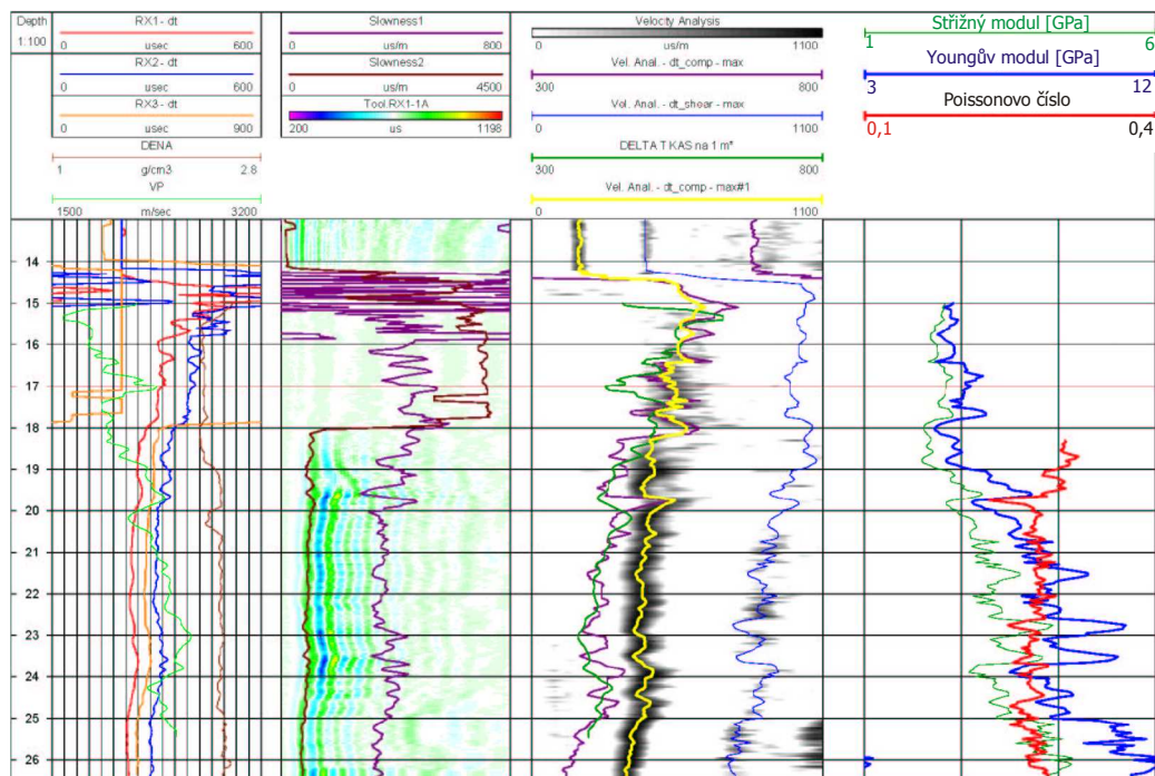
Obr. 4 Průběh strizného a Youngova modulu a Poissonova čísla podél osy vrtu (podle Aquatestu)
