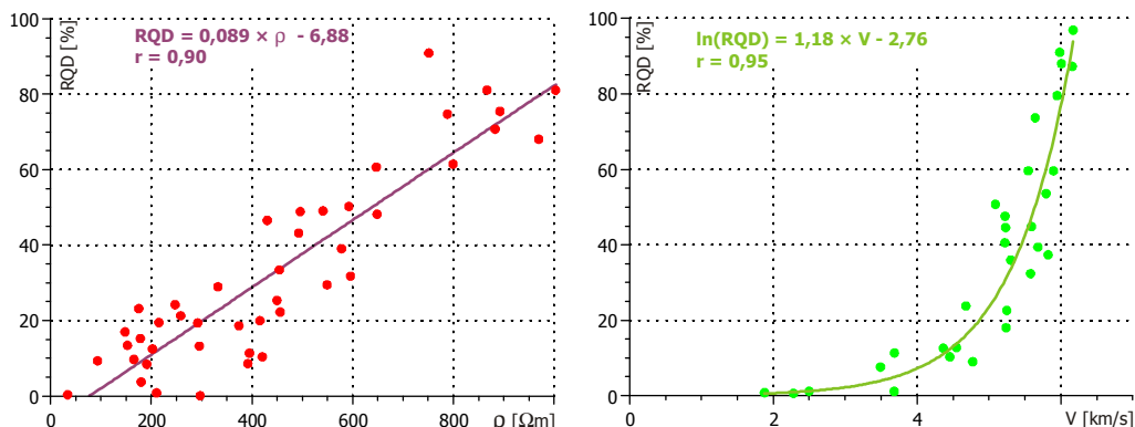
Obr. 1 Vztah měrného odporu, rychlosti podélných vln a RQD
